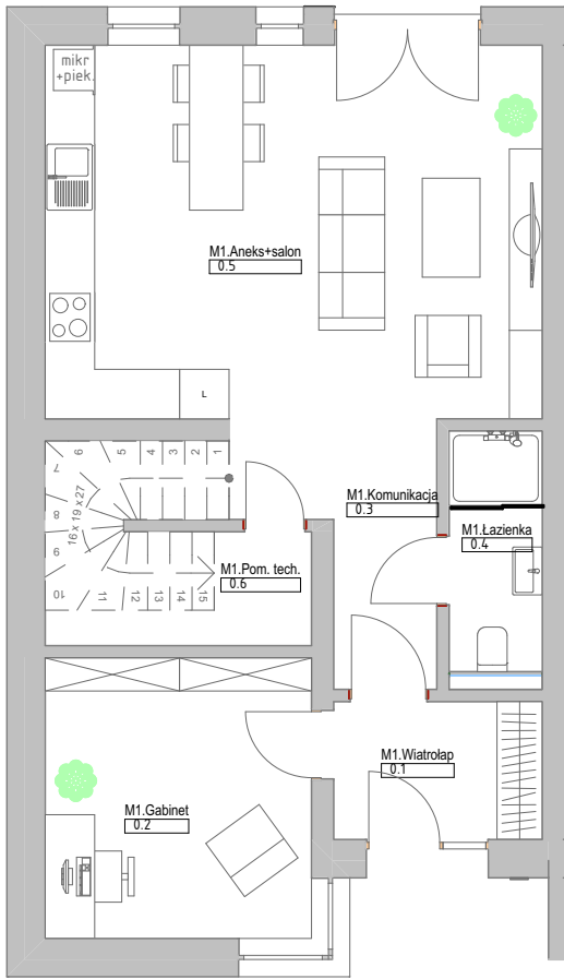
RZUT PARTERU
